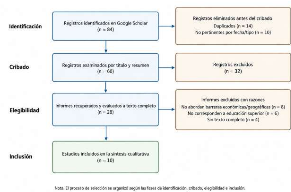
Figura 1. Diagrama de flujo PRISMA 2020 para la selección de estudios.
